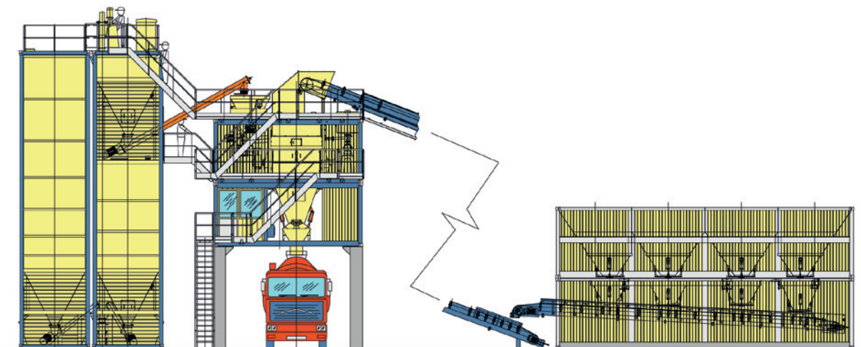
Planta de hormigón PHC-100 en contenedores ISO 20' estándar y 40' HC.
