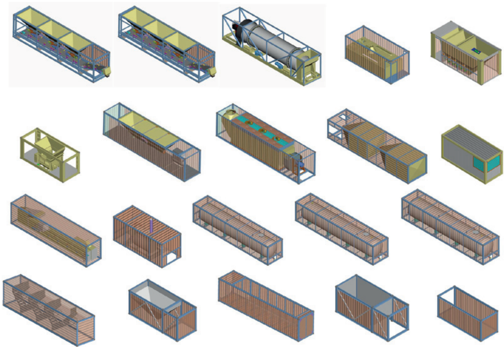
Configuración de contenedores para planta CM-160 con silo de aglomerado CSA-30.
