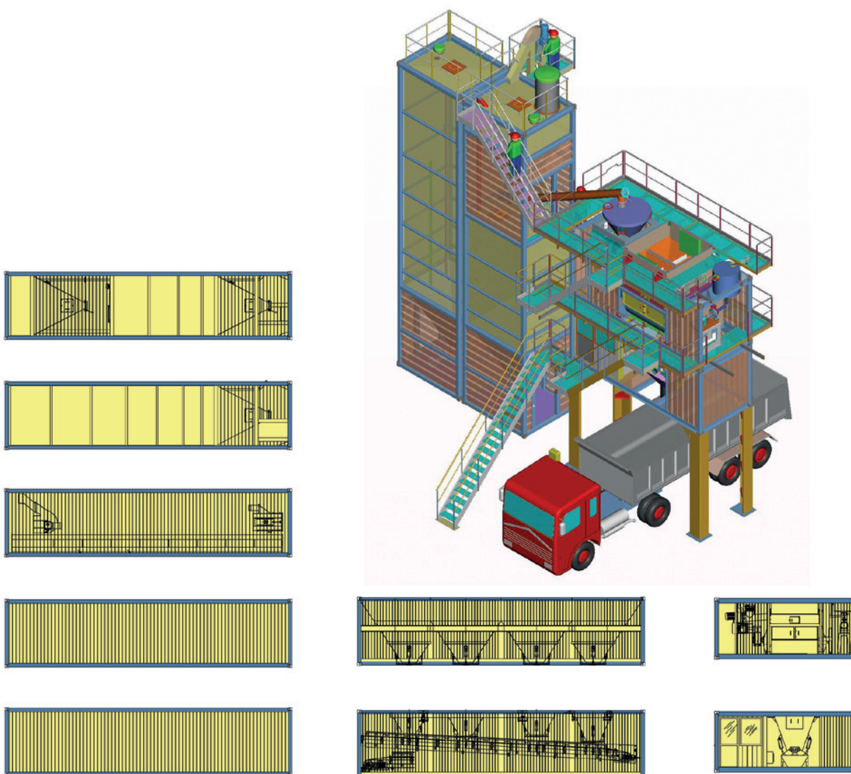
Configuración de contenedores para planta PHC-100.
