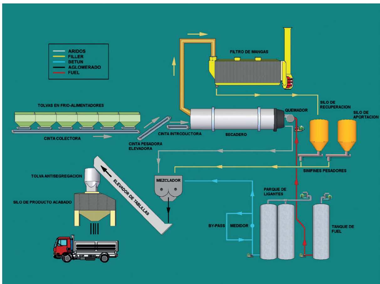
Diagrama de funcionamiento de plantas asfálticas continuas.
