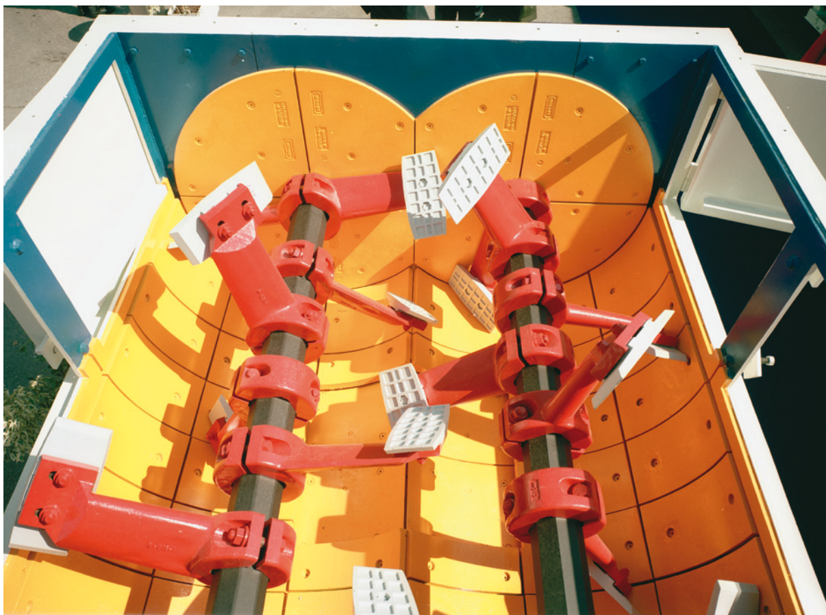
Vista del interior de la amasadora provista de palas, brazos y revestimientos recambiables de gran dureza.
