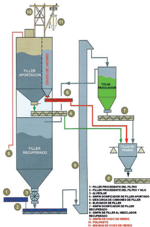
Equipo de incorporación de óxido de hierro.
