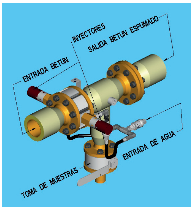
Equipo de espumación de betún BITFOAM para mezclas semi-calientes. Del tipo de rampa de espumación en línea. Dotado de sistema de espumación a presión constante independiente del caudal. La presión de pulverización es regulable.
