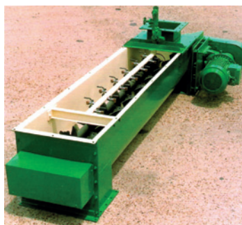
Humectador de polvo para fácil tratamiento del filler sobrante.
