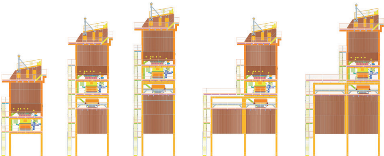
Configuración con distintos silos de aglomerado y con tolvas de áridos en caliente ampliadas
