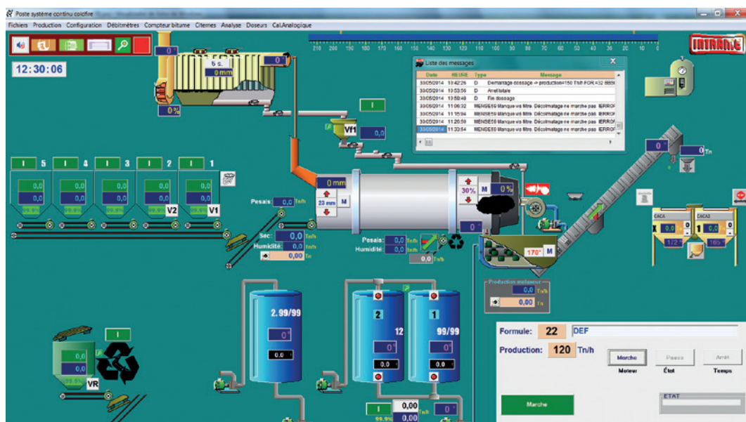
Sinóptico de control integral de planta continua.
