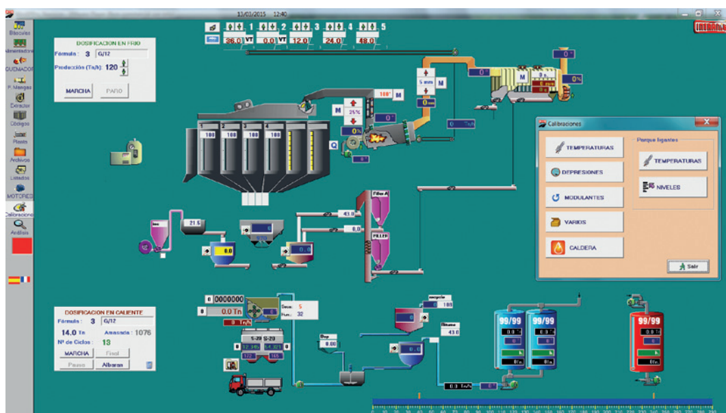
Sinóptico de control integral de planta discontinua.
