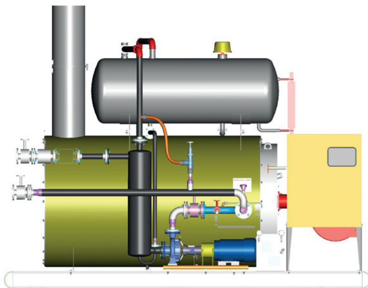
Gama INTRAME de Calderas de Fluido Térmico.
