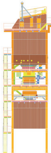
Torre S y Torre G, con la misma configuración y dibujadas con la misma escala
