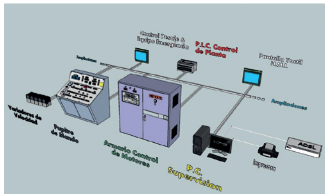
Moderna arquitectura de comunicaciones Ethernet/IP abierto y flexible.
