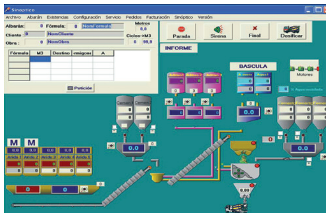
Pantalla con sinóptico de control integral de planta.
