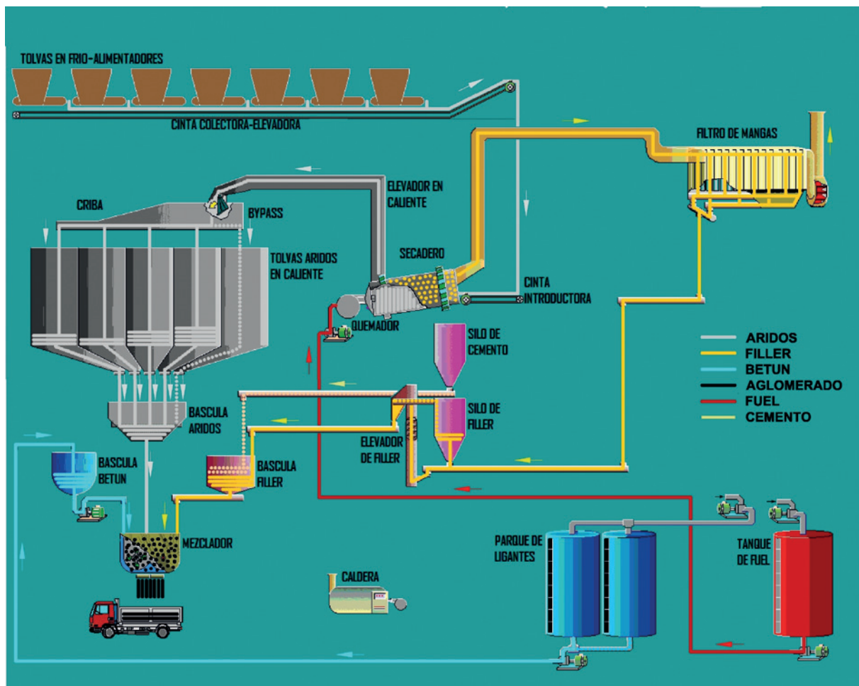
Diagrama de funcionamiento de plantas discontinuas.
