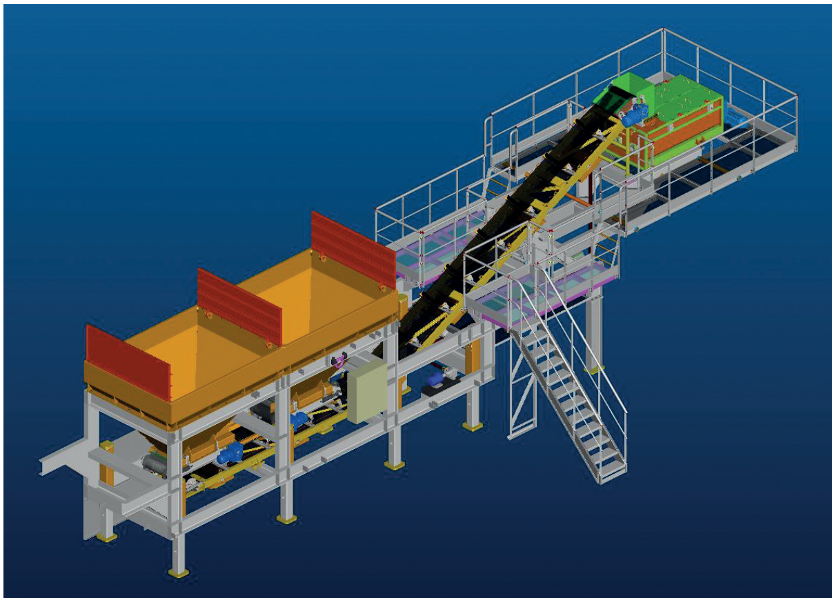
Planta de aglomerado en frío de 100 t/h.
