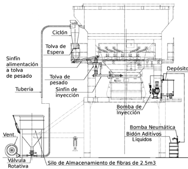
Equipo de Aditivo sólido tipo fibras y equipo de aditivo líquido.
