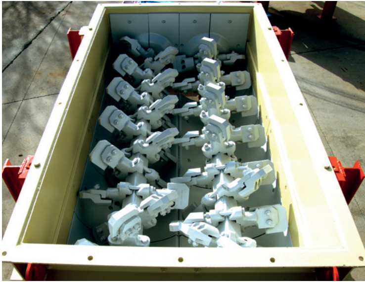
Mezclador continuo.
